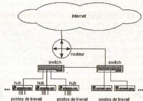
Un schéma d'un réseau LAN : Internet, un routeur et plein d'hôtes derrière, en interne.
