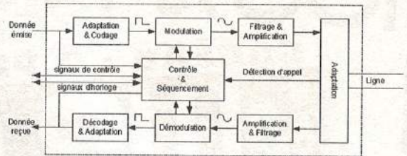
Pour les bricoleurs, le schéma fonctionnel complet du modem : ses entrées/sorties, ses calculs de synchronisation...
