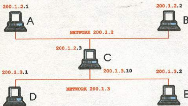
La machine du milieu est un routeur. C'est le point central entre l'intérieur et l'extérieur.
